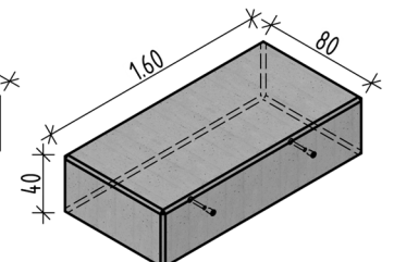
Typ 100-4 glatt unten
