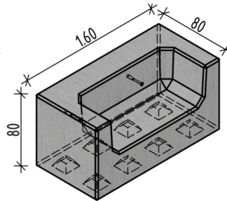
Typ 3 mit Noppen unten
