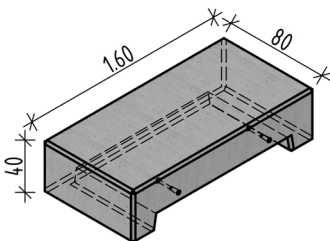
Typ 100 mit Vertiefung
