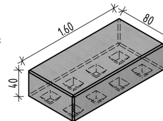
Typ 100-3 mit Noppen unten
