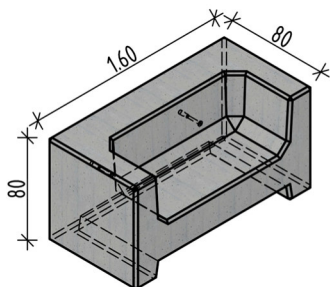
Typ 1 mit Vertiefung
