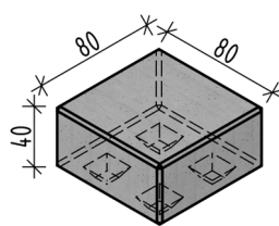
Typ 200-3 mit Noppen unten
