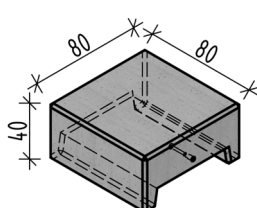
Typ 200-2 mit Aussparung
