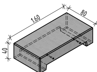
Typ 100-2 mit Aussparung
