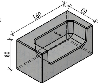
Typ 4 glatt unten
