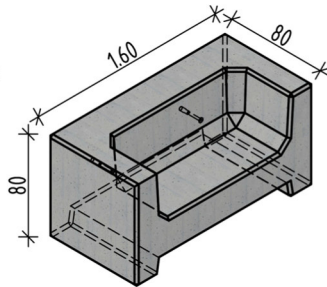
Typ 2 mit Aussparung
