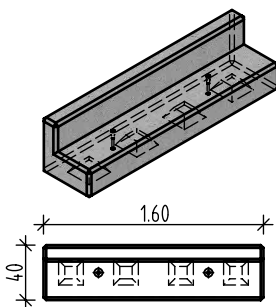
Typ 40-8
