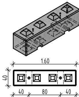
Typ 40-4
