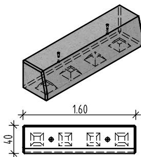
Typ 40-9
