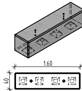
Typ 40-6
