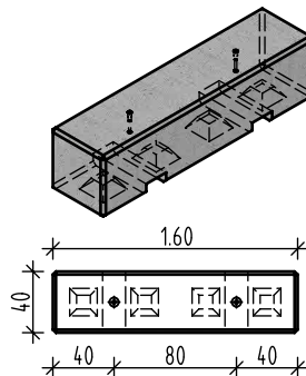
Typ 40-5
