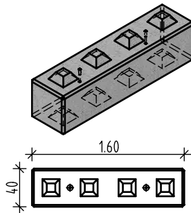
Typ 40
