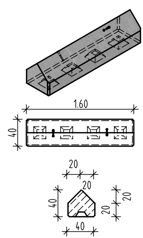
Typ 40-7
